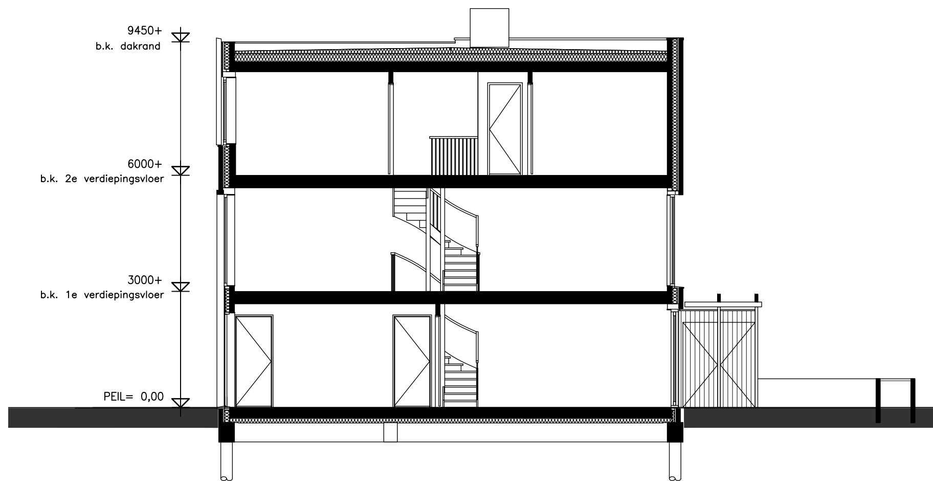
langsdoorsnede
