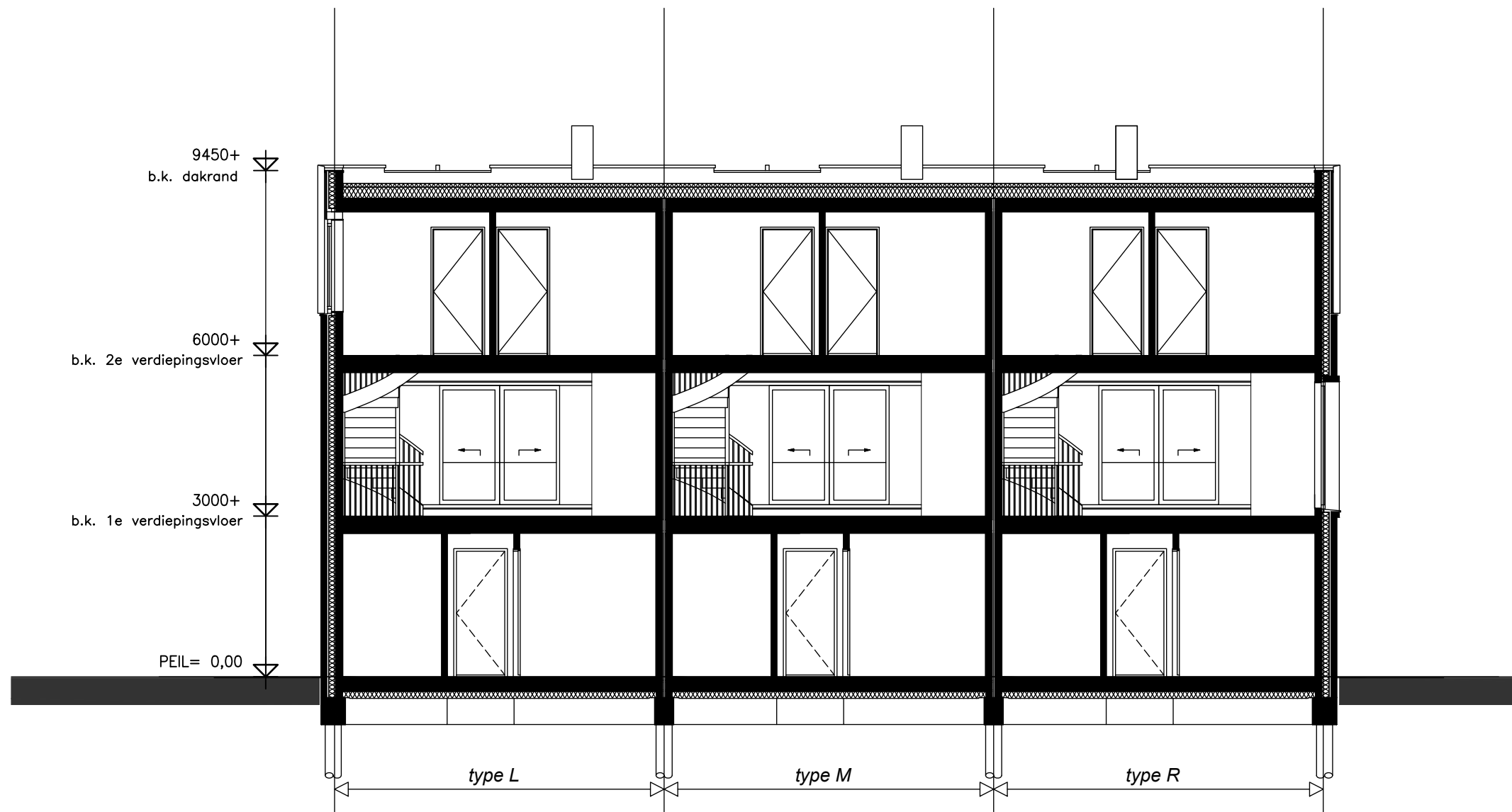
dwarsdoorsnede
